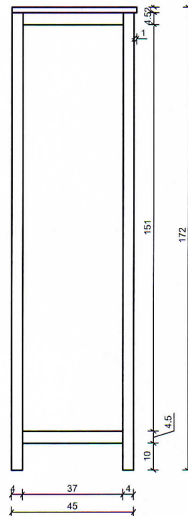
BOČNI POGLED
