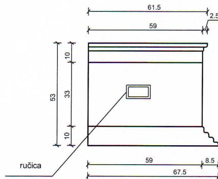
BOČNI POGLED
