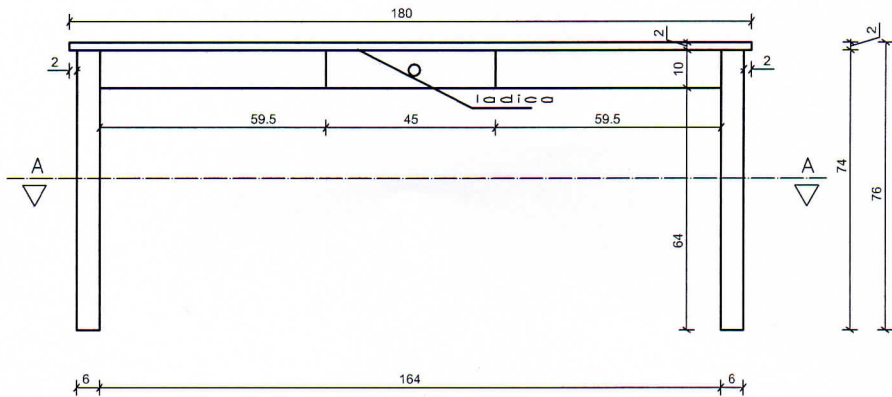
POGLED
