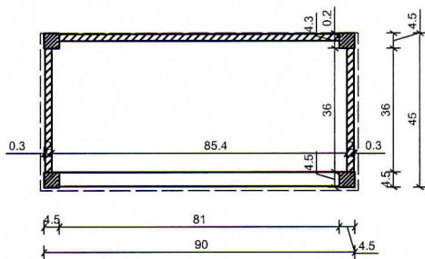
TLOCRT NIVO A-A
