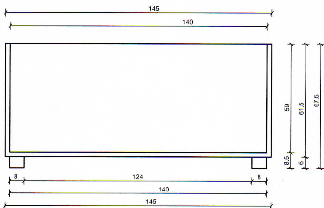
TLOCRT
