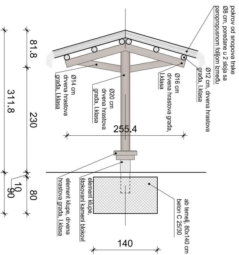
POPREČNI PRESJEK MJ 1:50
